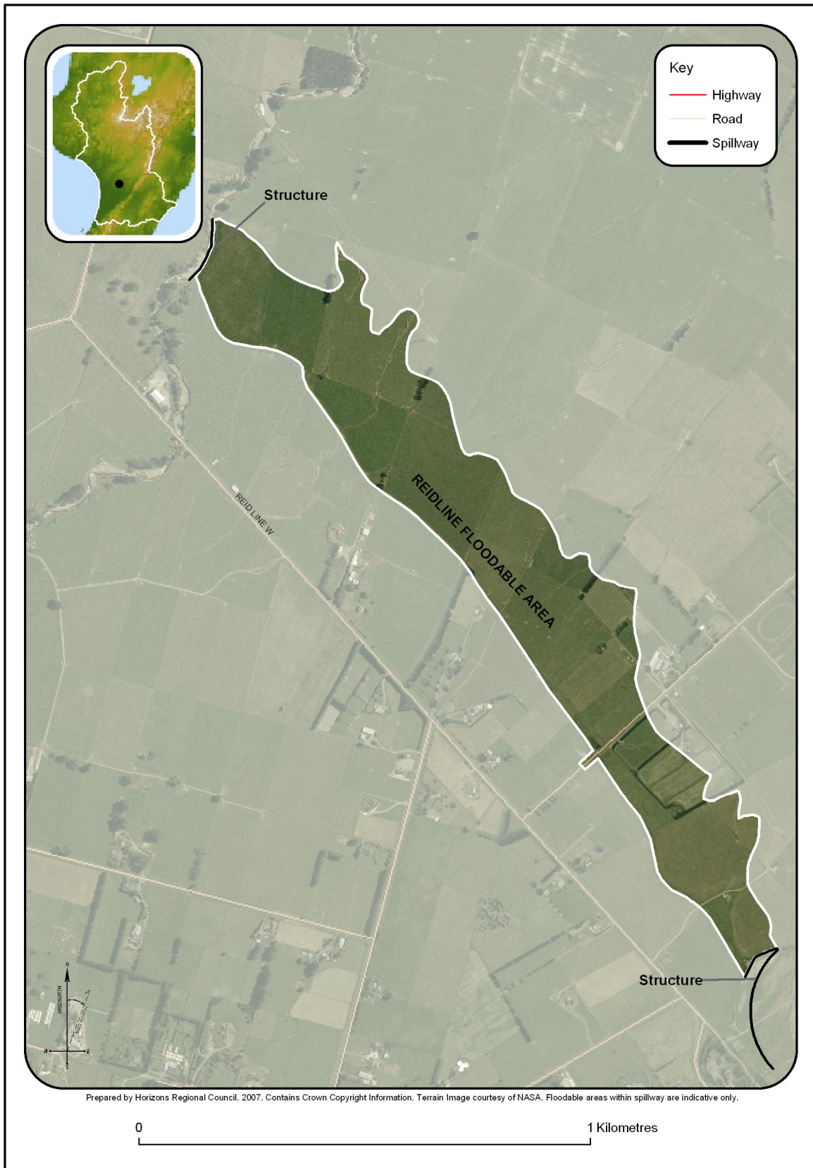
Figure I:4 Makino Spillway
