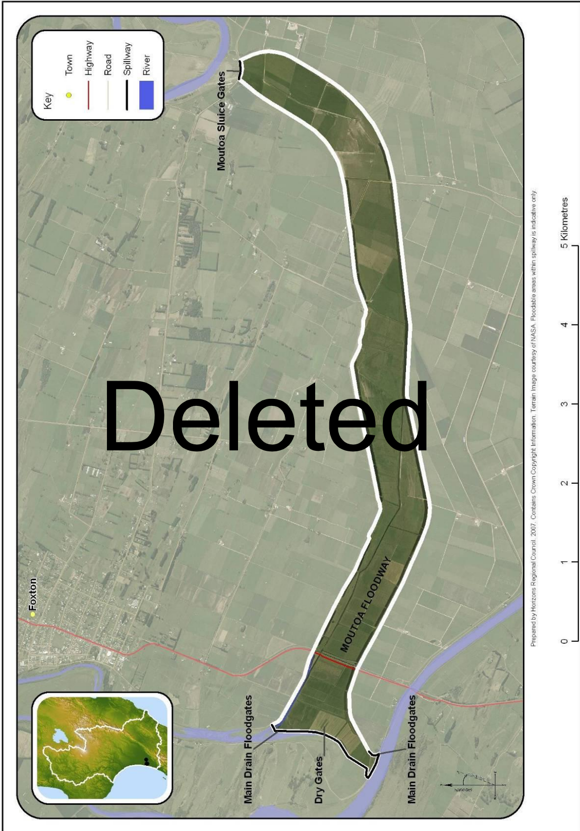
Figure I:2— Moutoa Spillway
